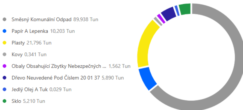
Sumarizační graf
